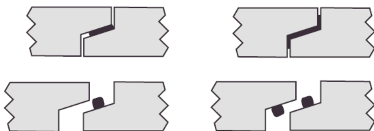
ÉTANCHÉITÉ SUR PONCEAU RECTANGULAIRE (BUTYL 1" )
