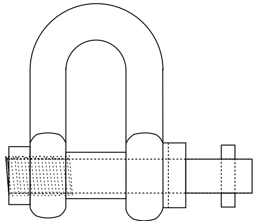
SYSTÈME DE LEVAGE POUR BASES DE PUISARDS DE 600Ø@900Ø & OU ANNEAUX ET TÊTES DE REGARDS ET PUISARDS DE 600Ø@900Ø
