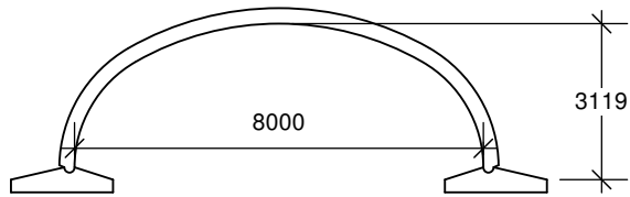
TYPE 1 aire hydraulique 20,02 m 2 rayon hydraulique 1,052 m
