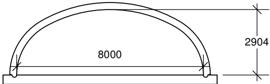
TYPE 6 rayon hydraulique 29,04 m 2 rayon hydraulique 0,968 m
