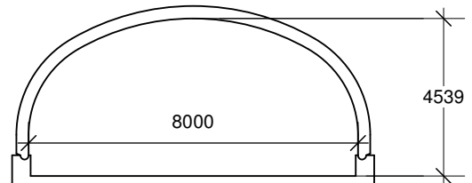
TYPE 5 rayon hydraulique 31,20 m 2 rayon hydraulique 1,410 m
