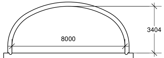
TYPE 7 rayon hydraulique 22,33 m 2 rayon hydraulique 1,118 m
