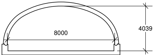
TYPE 4 rayon hydraulique 29,13 m 2 rayon hydraulique 1,288 m
