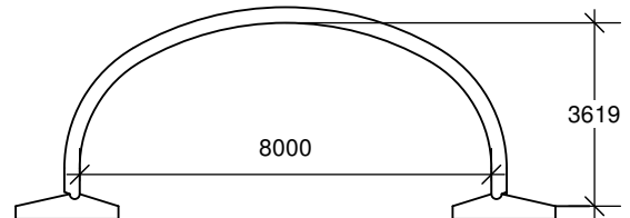
TYPE 2 rayon hydraulique 24,03 m 2 rayon hydraulique 1,199 m
