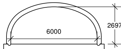
TYPE 7 aire hydraulique 13,38 m 2 rayon hydraulique 0,878 m
