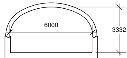
TYPE 4 aire hydraulique 16,90 m 2 rayon hydraulique 1,031 m
