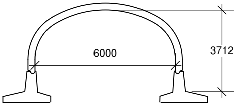
TYPE 3 aire hydraulique 19,41 m 2 rayon hydraulique 1,143 m
