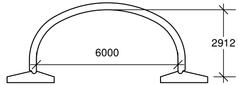
TYPE 2 aire hydraulique 14,56 m 2 rayon hydraulique 0,951 m
