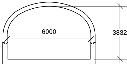
TYPE 5 aire hydraulique 19,90 m 2 rayon hydraulique 1,144 m
