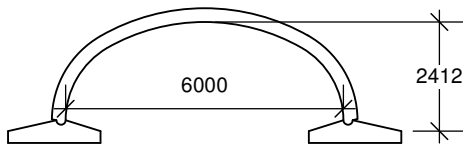
TYPE 1 aire hydraulique 5,04 m 2 rayon hydraulique 0,583 m
