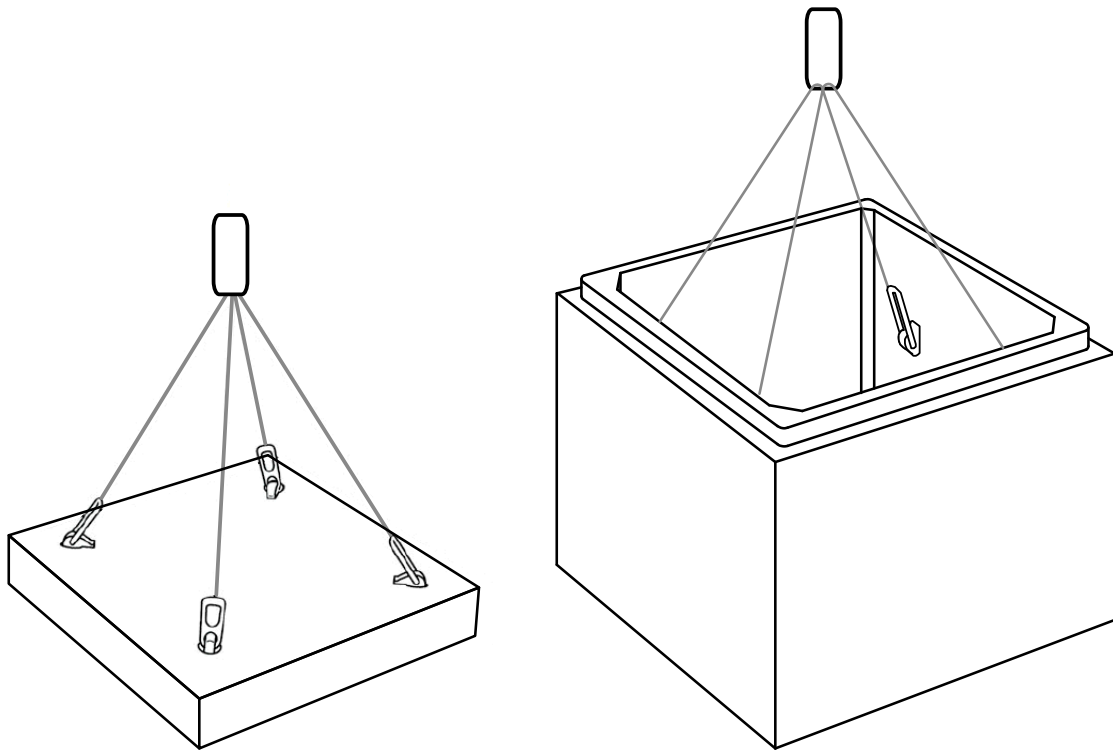
EXEMPLE D'INSTALLATION
