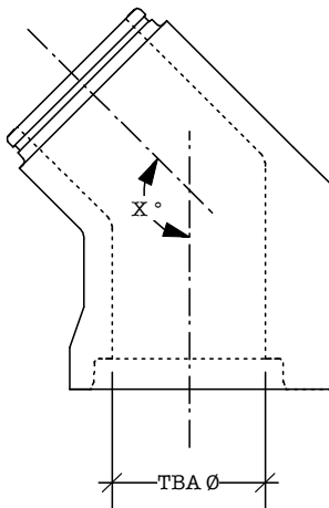
COUDE 250Ø @ 600Ø X 1 M.LIN
