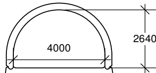
TYPE 2 aire hydraulique 8,75 m.c. rayon hydraulique 0,766 m
