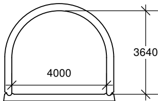
TYPE 4 aire hydraulique 12,75 m.c. rayon hydraulique 0,950 m
