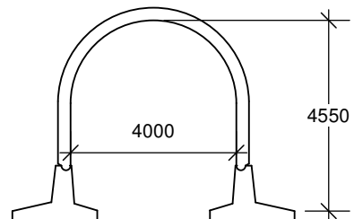
TYPE 9 aire hydraulique 16,20 m.c. rayon hydraulique 1,076 m
