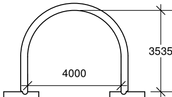
TYPE 8 aire hydraulique 12,40 m.c. rayon hydraulique 0,929 m
