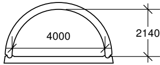
TYPE 1 aire hydraulique 6,75 m.c. rayon hydraulique 0,647 m
