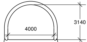
TYPE 3 aire hydraulique 10,75 m.c. rayon hydraulique 0,866 m
