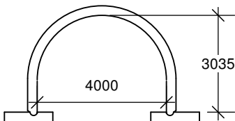
TYPE 7 aire hydraulique 10,40 m.c. rayon hydraulique 0,843 m
