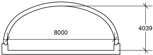
TYPE 4 rayon hydraulique 29,13 m.c. rayon hydraulique 1,288 m
