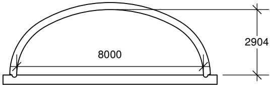
TYPE 6 rayon hydraulique 29,04 m.c. rayon hydraulique 0,968 m
