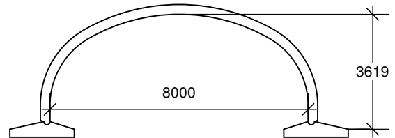
TYPE 2 rayon hydraulique 24,03 m.c. rayon hydraulique 1,199 m
