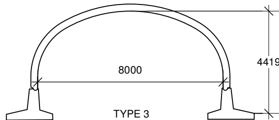
TYPE 3 aire hydraulique 30,48 m.c. rayon hydraulique 1,404 m
