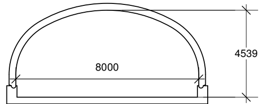
TYPE 5 rayon hydraulique 31,20 m.c. rayon hydraulique 1,410 m
