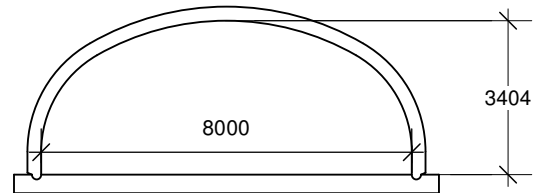
TYPE 7 rayon hydraulique 22,33 m.c. rayon hydraulique 1,118 m
