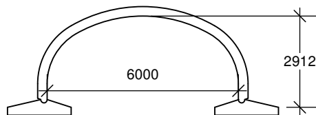
TYPE 2 aire hydraulique 14,56 m.c. rayon hydraulique 0,951 m
