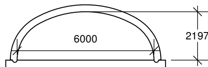
TYPE 6 aire hydraulique 10,38 m.c. rayon hydraulique 0,728 m
