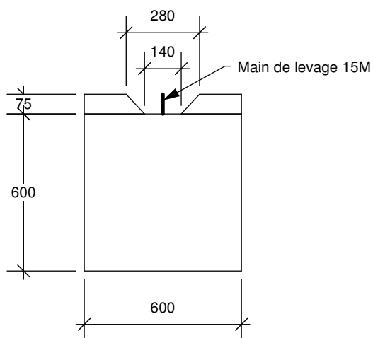
Vue élévation
