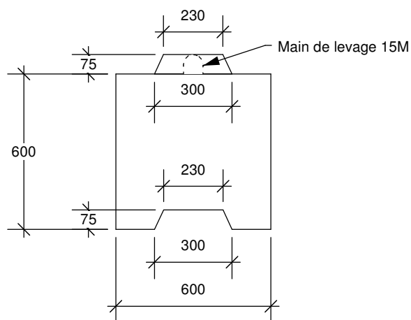
Vue latérale
